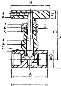
KE-8311A
